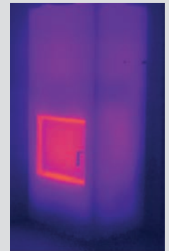
3 Std. nach dem Anheizen Durchschnittliche Oberflächentemperatur 37 °C
